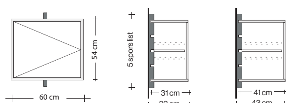
Konsoller høyde 54 cm - Dybde 31/41cm Minimum listlengde = 5 spor
