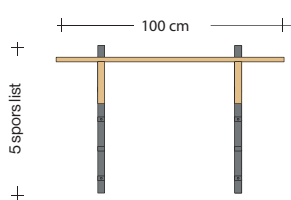
Oppriss front - Åpent
